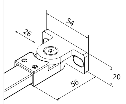
b WSPORNIK
