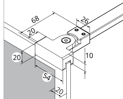
d WSPORNIK
