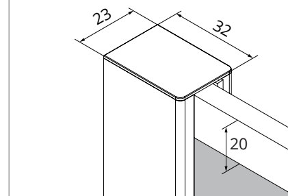
b WSPORNIK
