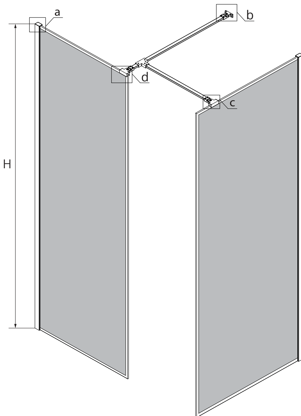
b WSPORNIK
