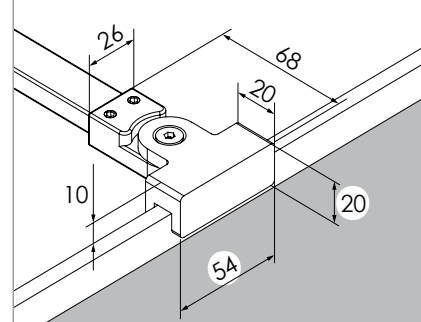
c WSPORNIK
